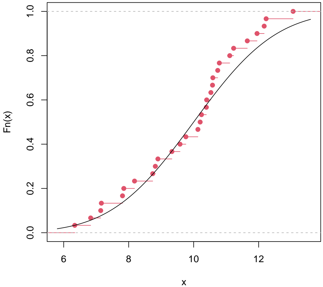
ecdf(X)
